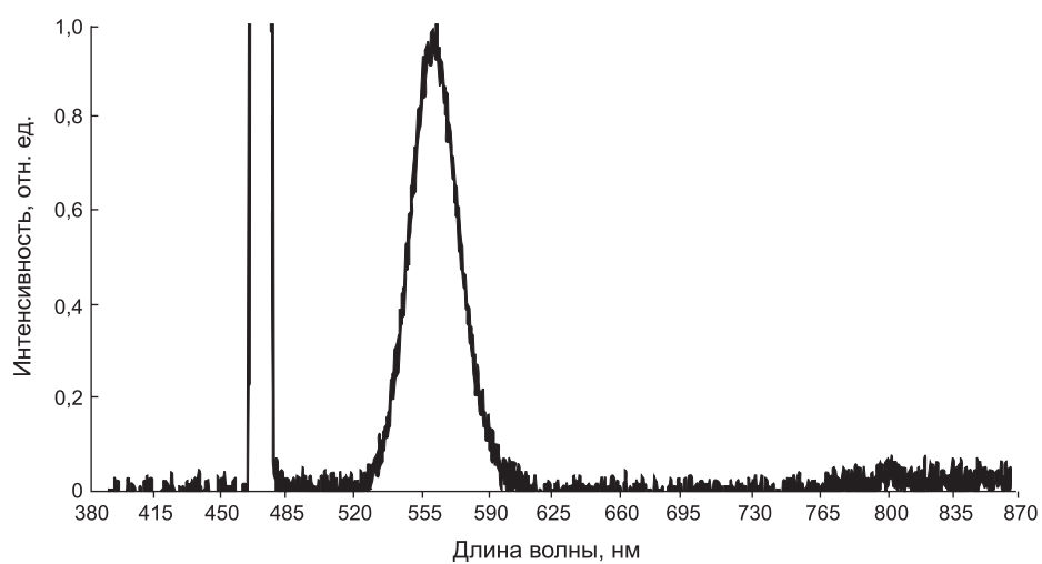
Рис. 4. Спектры возбуждения и флюоресценции наноконплексов с квантовыми точками Qtracker 565.
