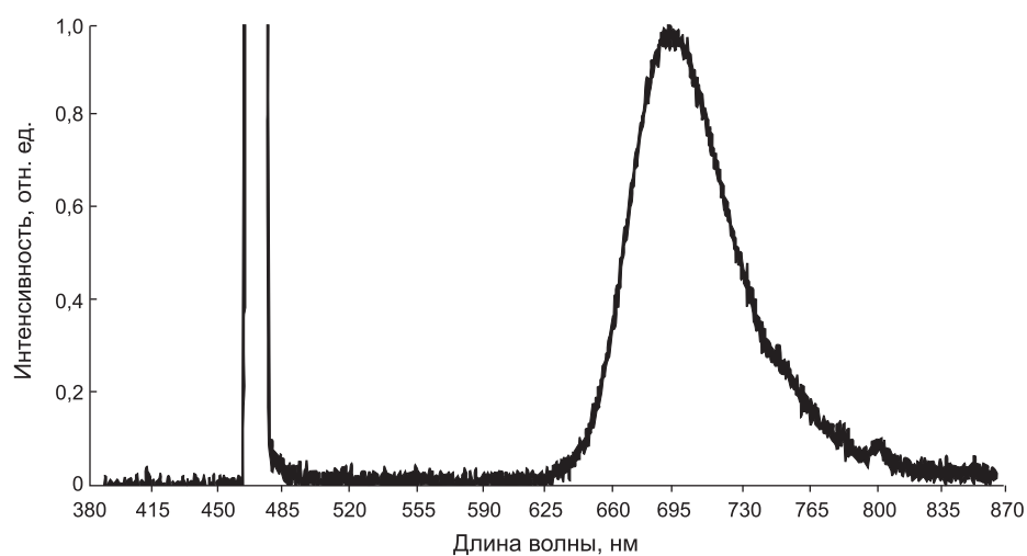
Рис. 5. Спектры возбуждения и флюоресценции наноконплексов с квантовыми точками Qtracker 705.
